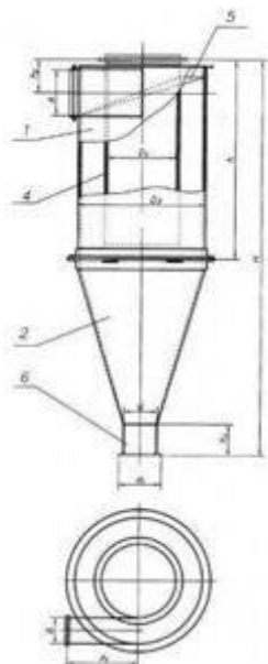
ЦИКЛОН ЛИОТ № 1 – 4
