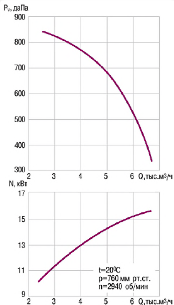
Аэродинамические характеристики ВПЗ № 3,6/650
