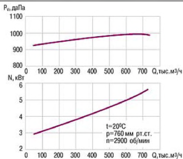
Аэродинамические характеристики ВПЗ № 3,6/650
